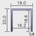
107- 20x19x1,4 aluminum anodise
